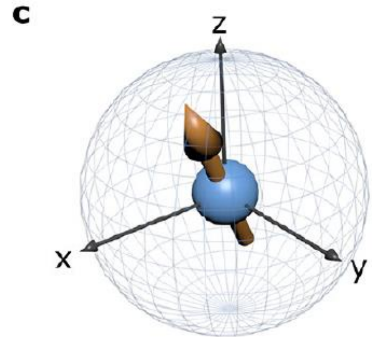
n=3 (3D-Heisenberg)
